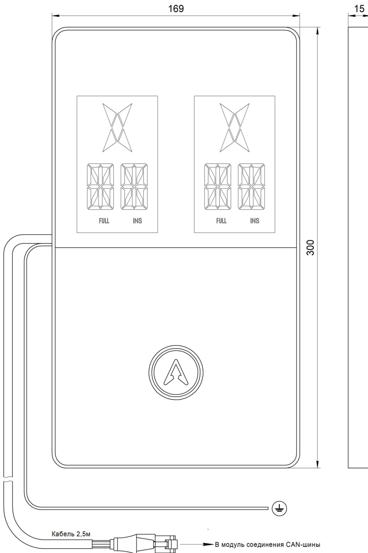
Рис.1 Внешний вид Вызывной пост ОНИКС (жгут RJ45) НШЕК.468381.119
